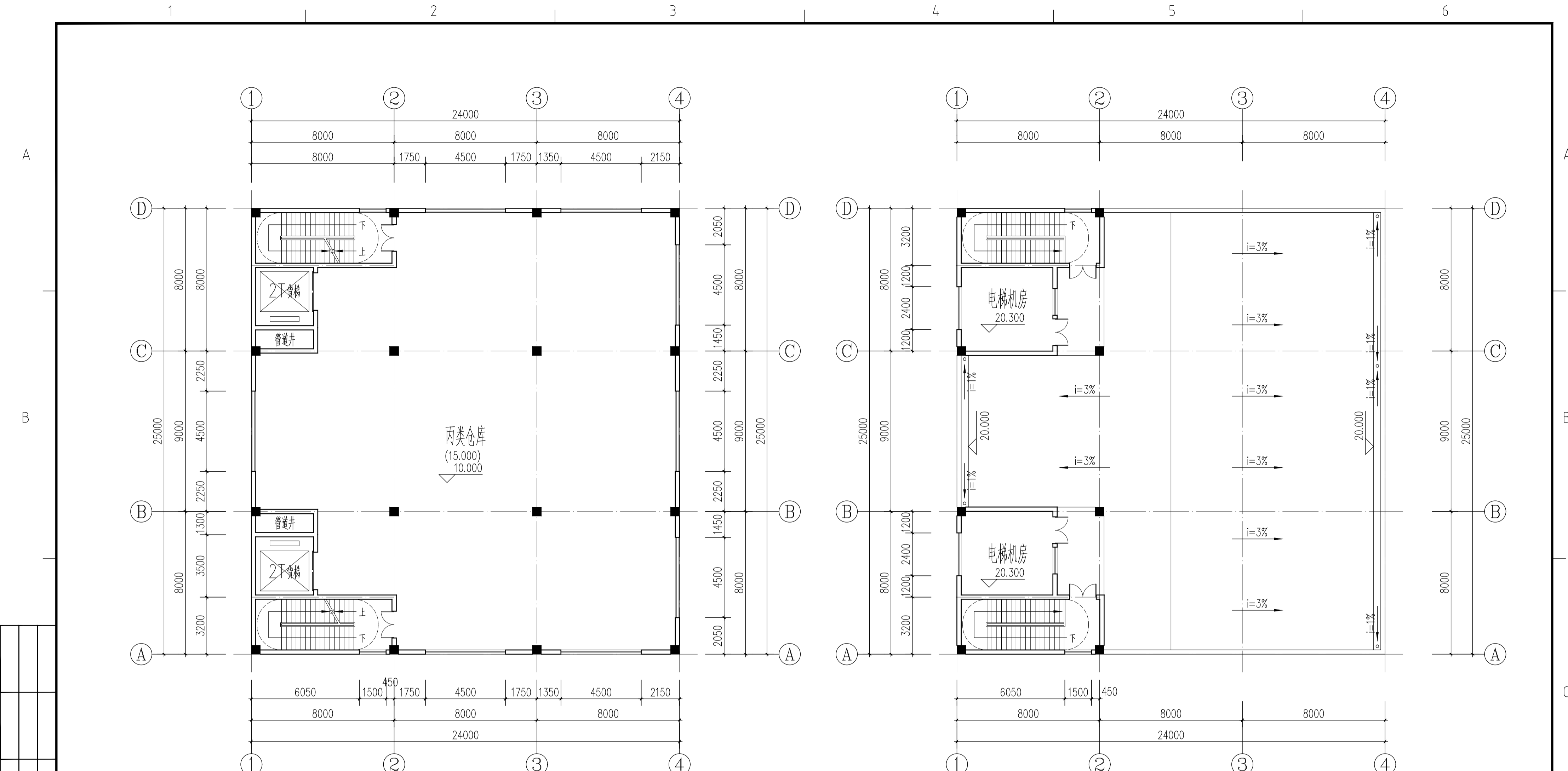
三、四层平面布置图 1:150
