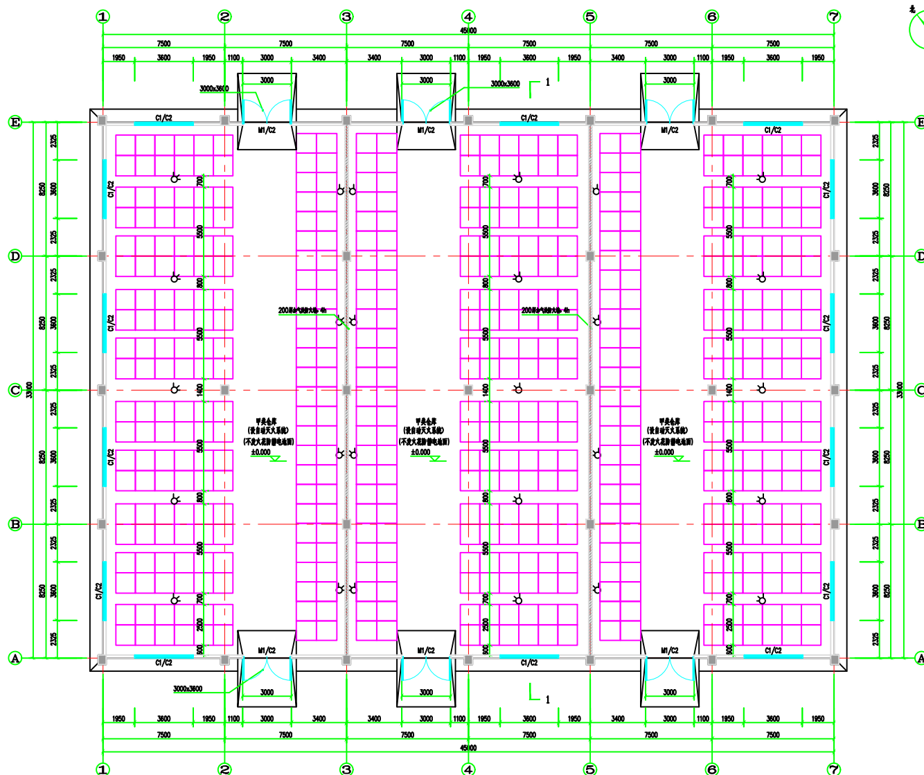
首层平面图 1:100
