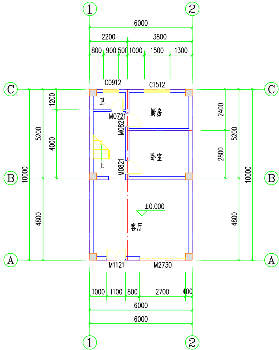
首层平面图1:100
