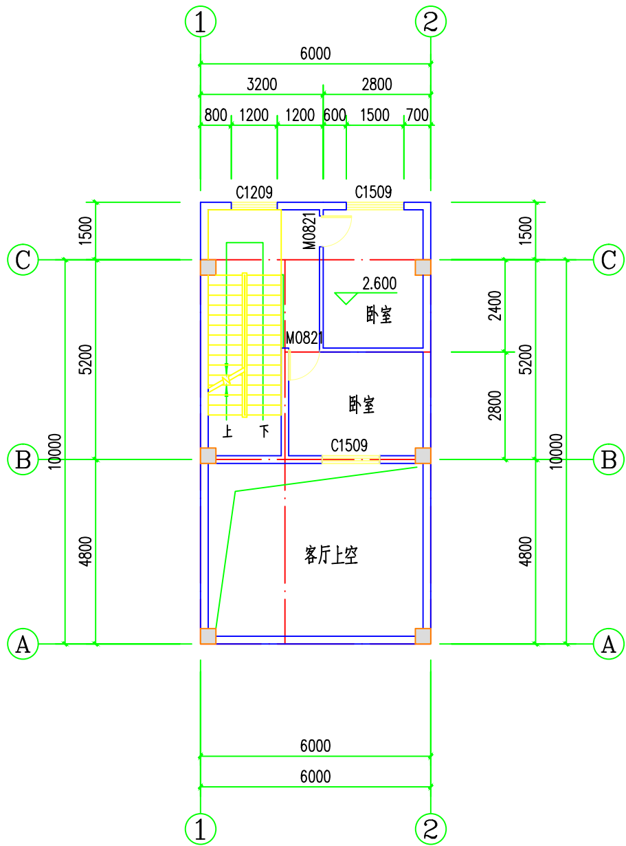
夹层平面图 1:100
