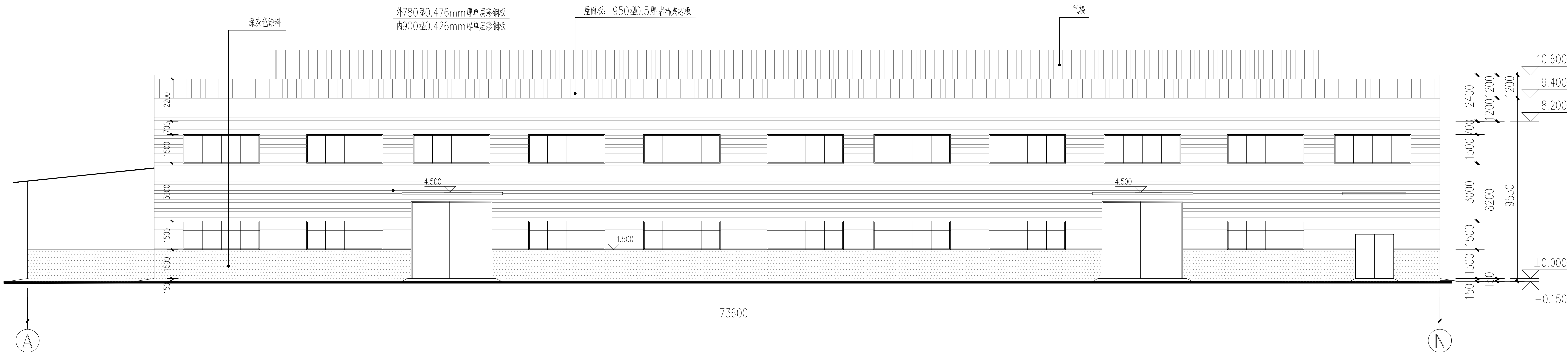
A~N轴立面图 1:120
