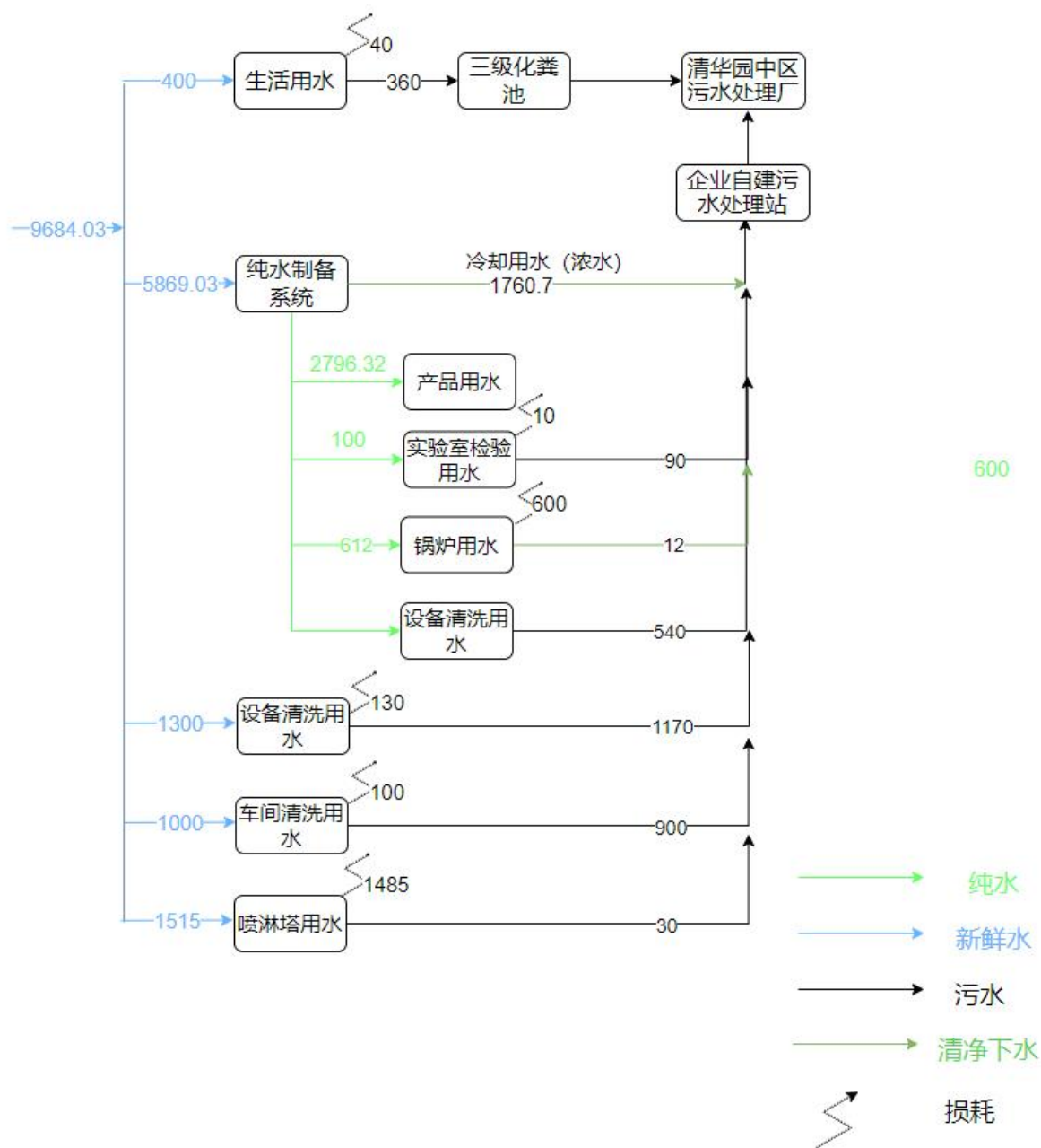
图 2-2 本项目水平衡图 (单位: \text{m}^3/\text{a} )
