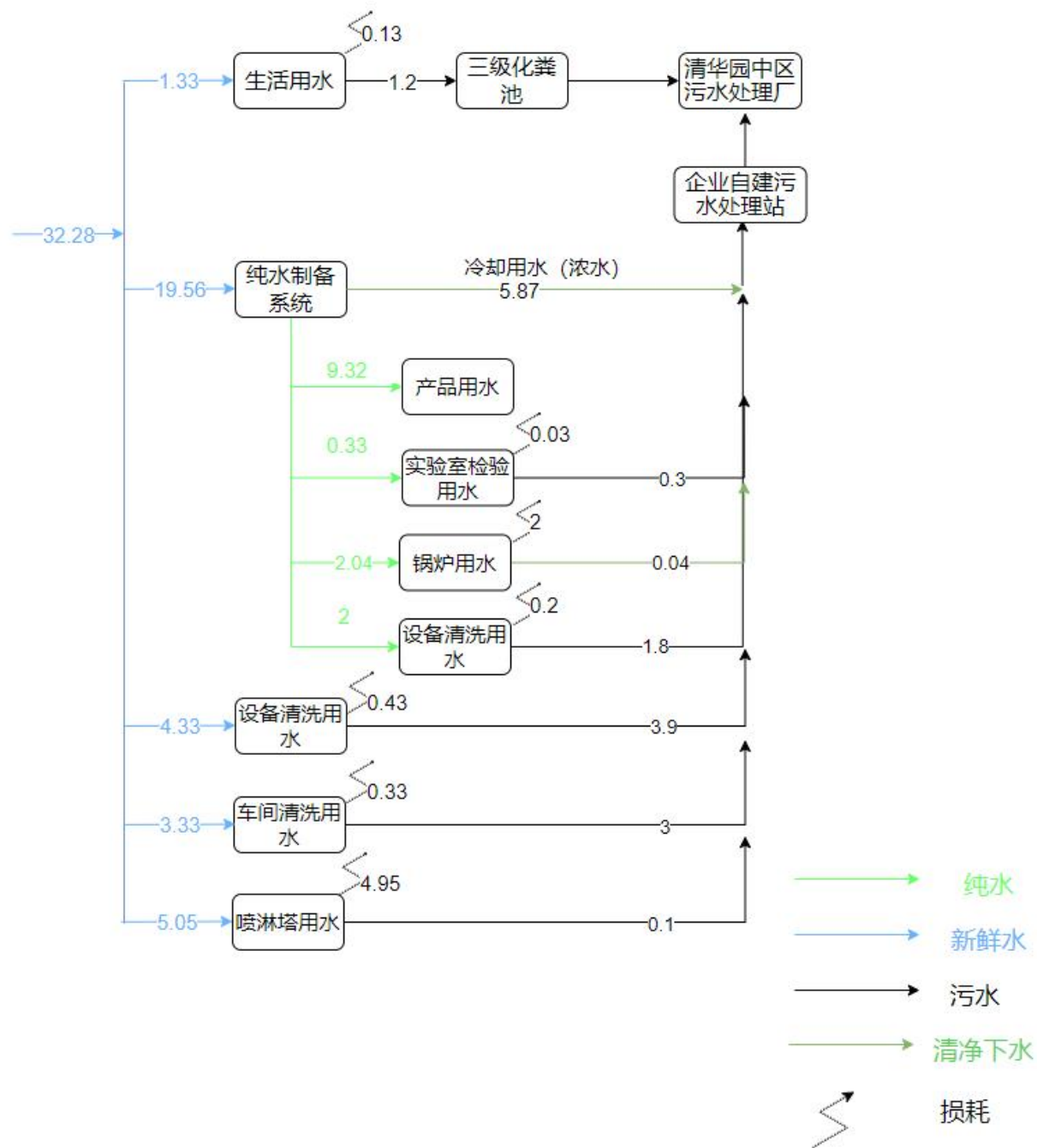
图 2-3 本项目水平衡图 (单位: m³/d)
