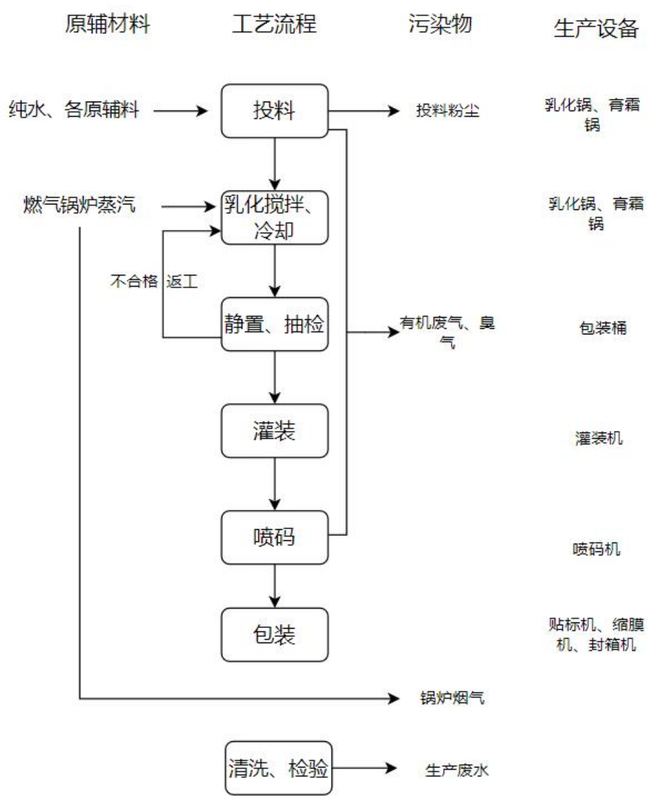
图 2-4 本项目生产工艺流程图
