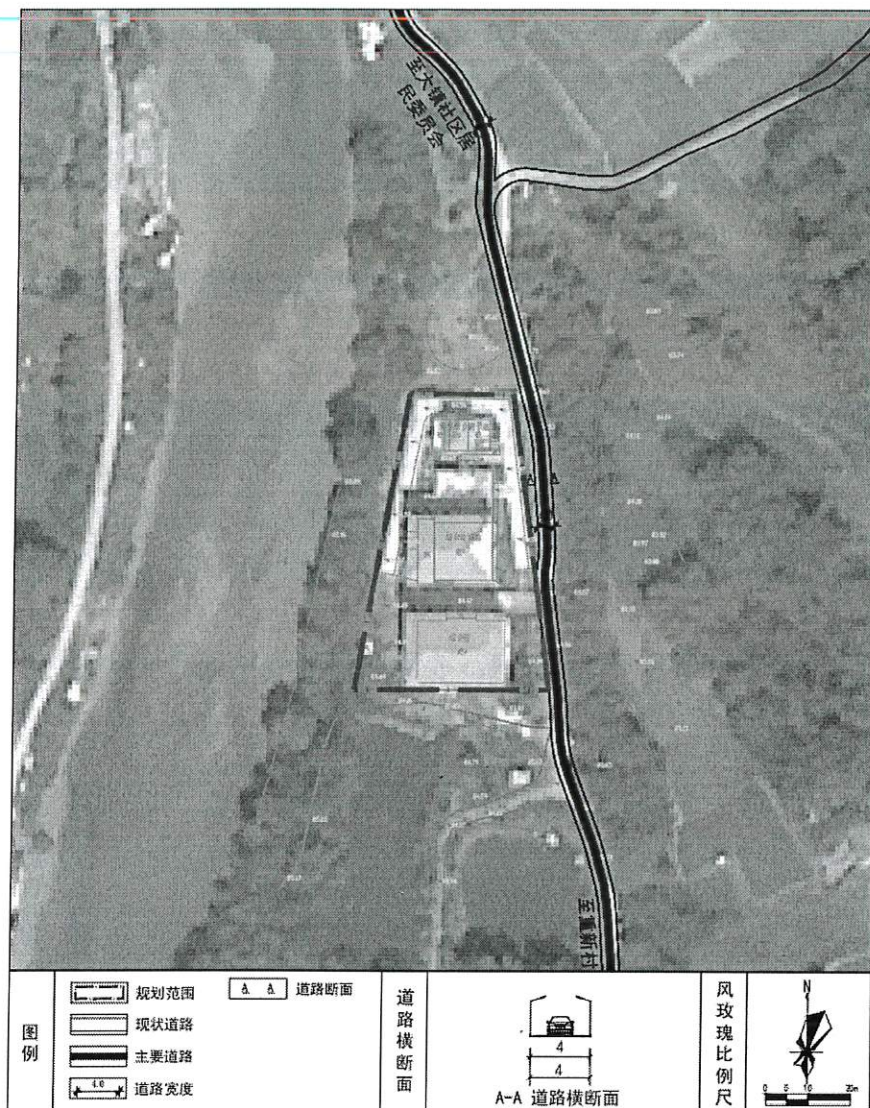
道路交通系统规划图
