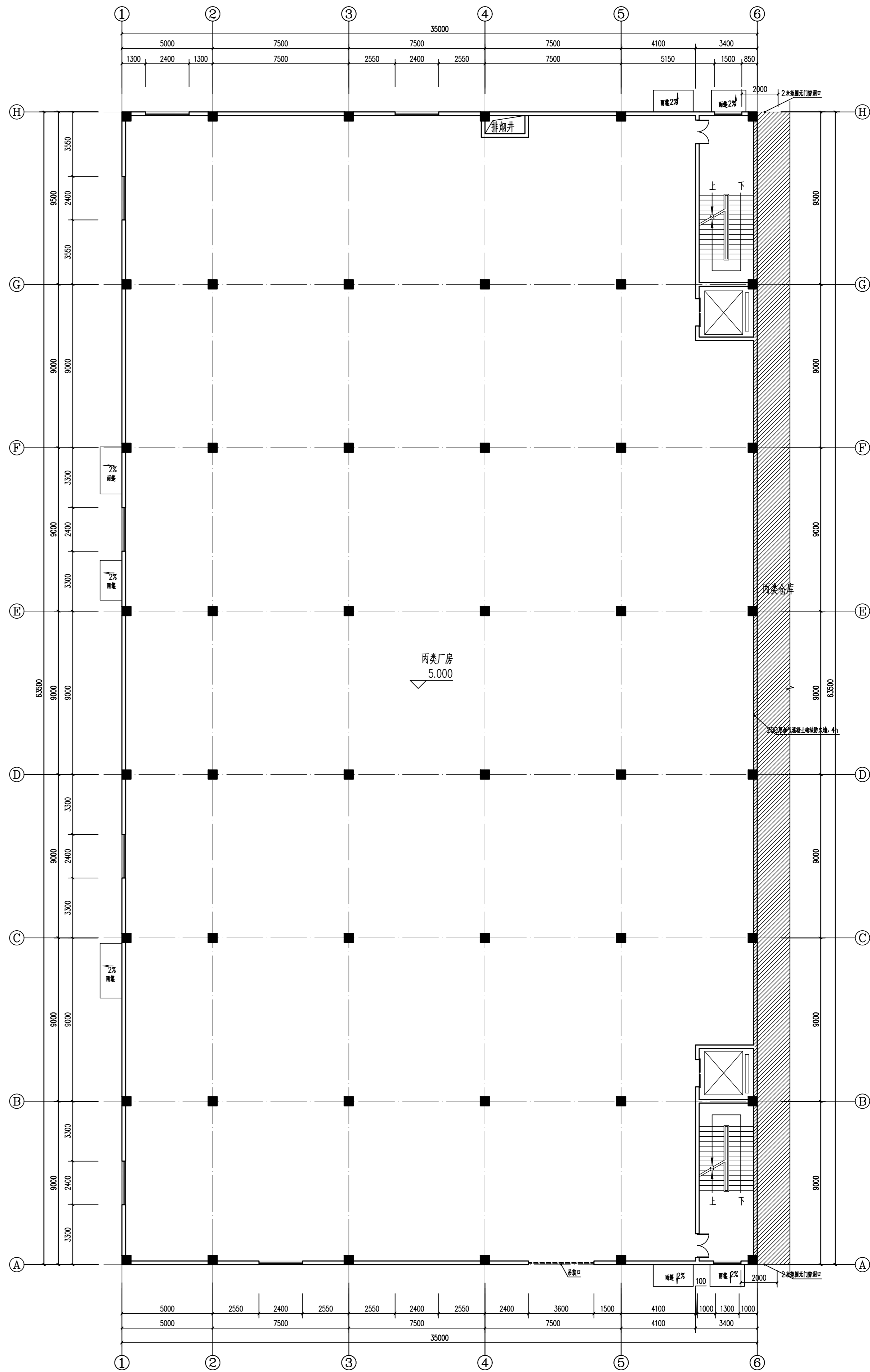
二层平面图 1:100
