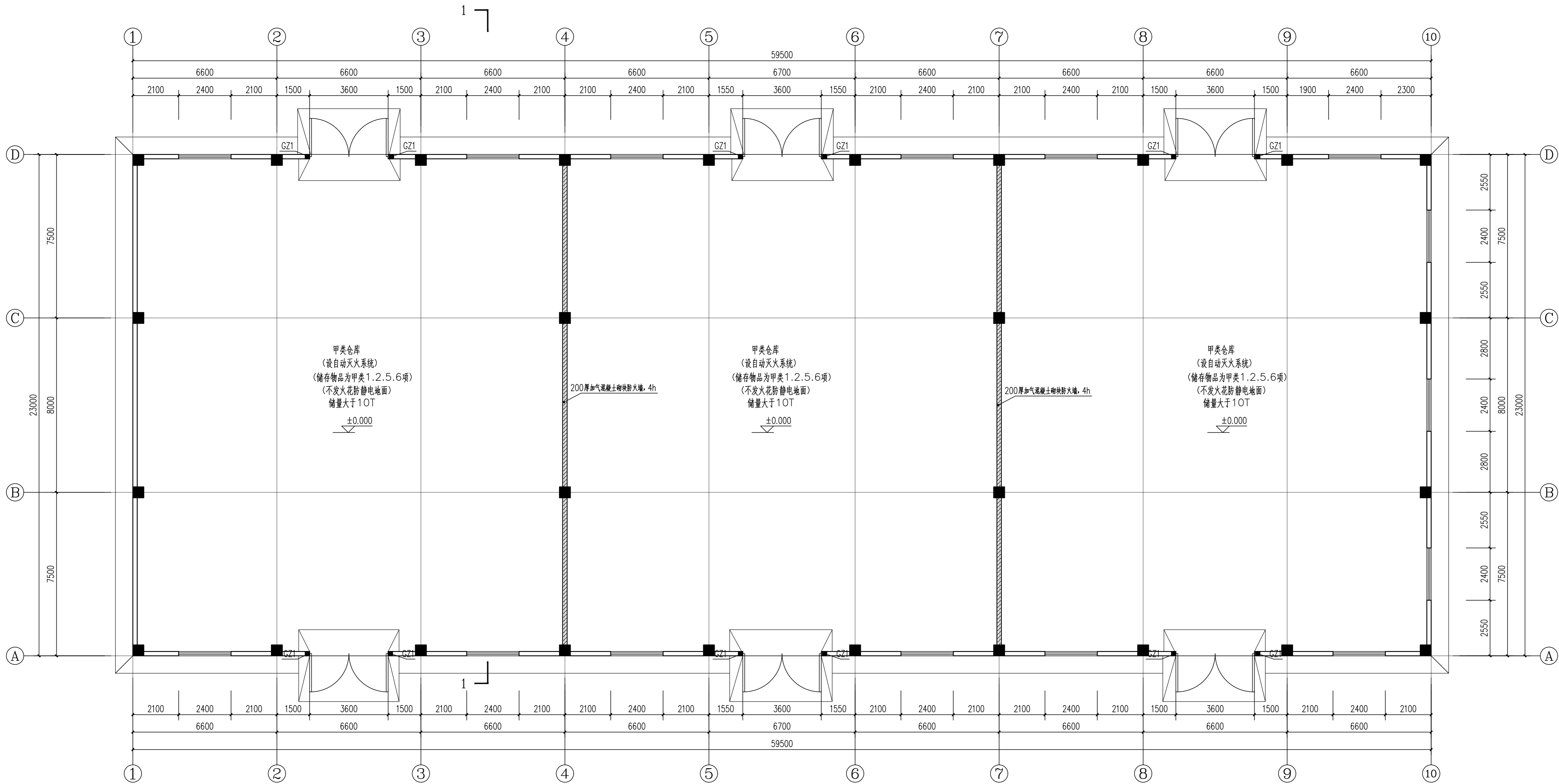
首层平面图 1:100
