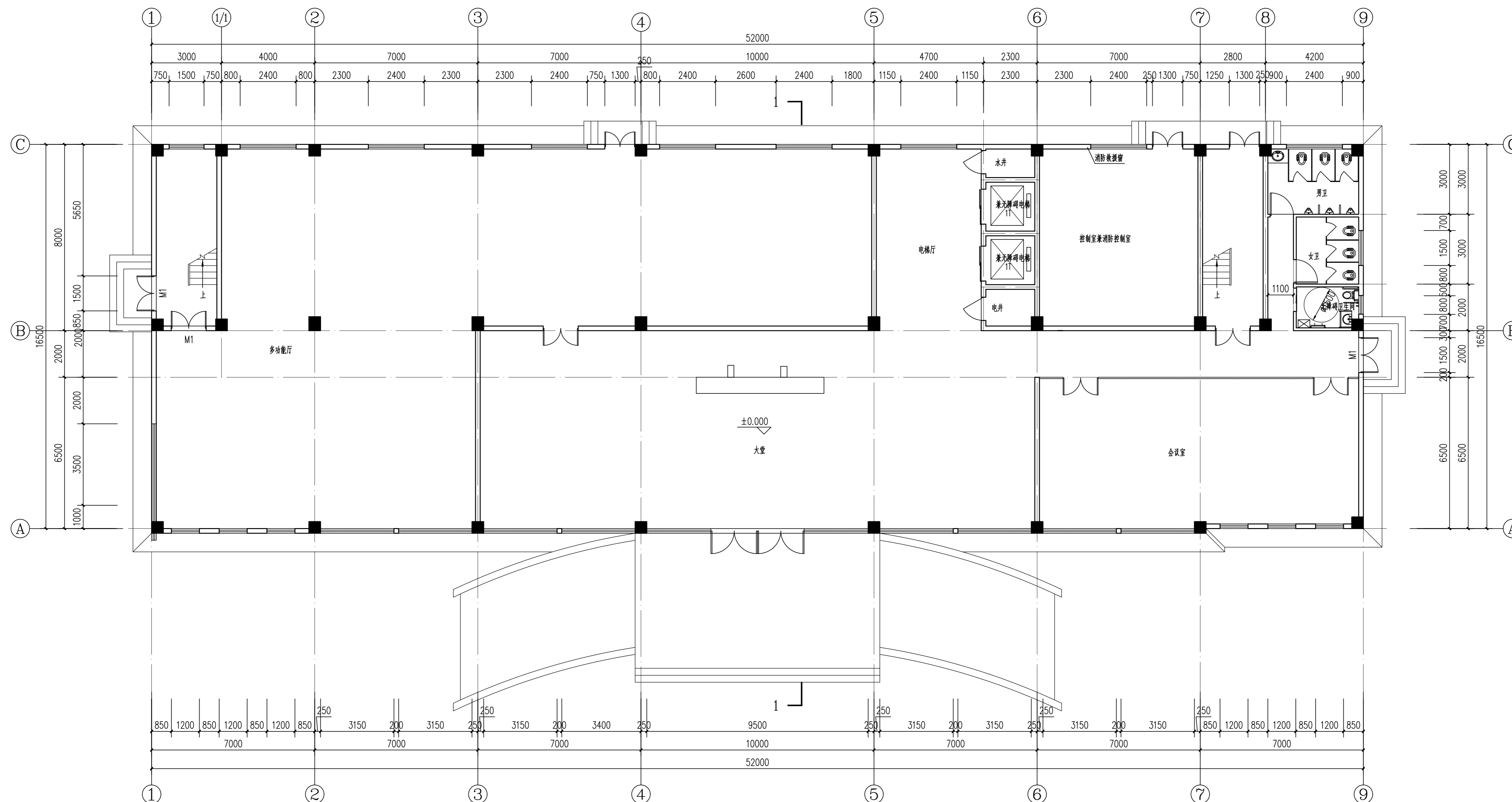
首层平面图 1:100
