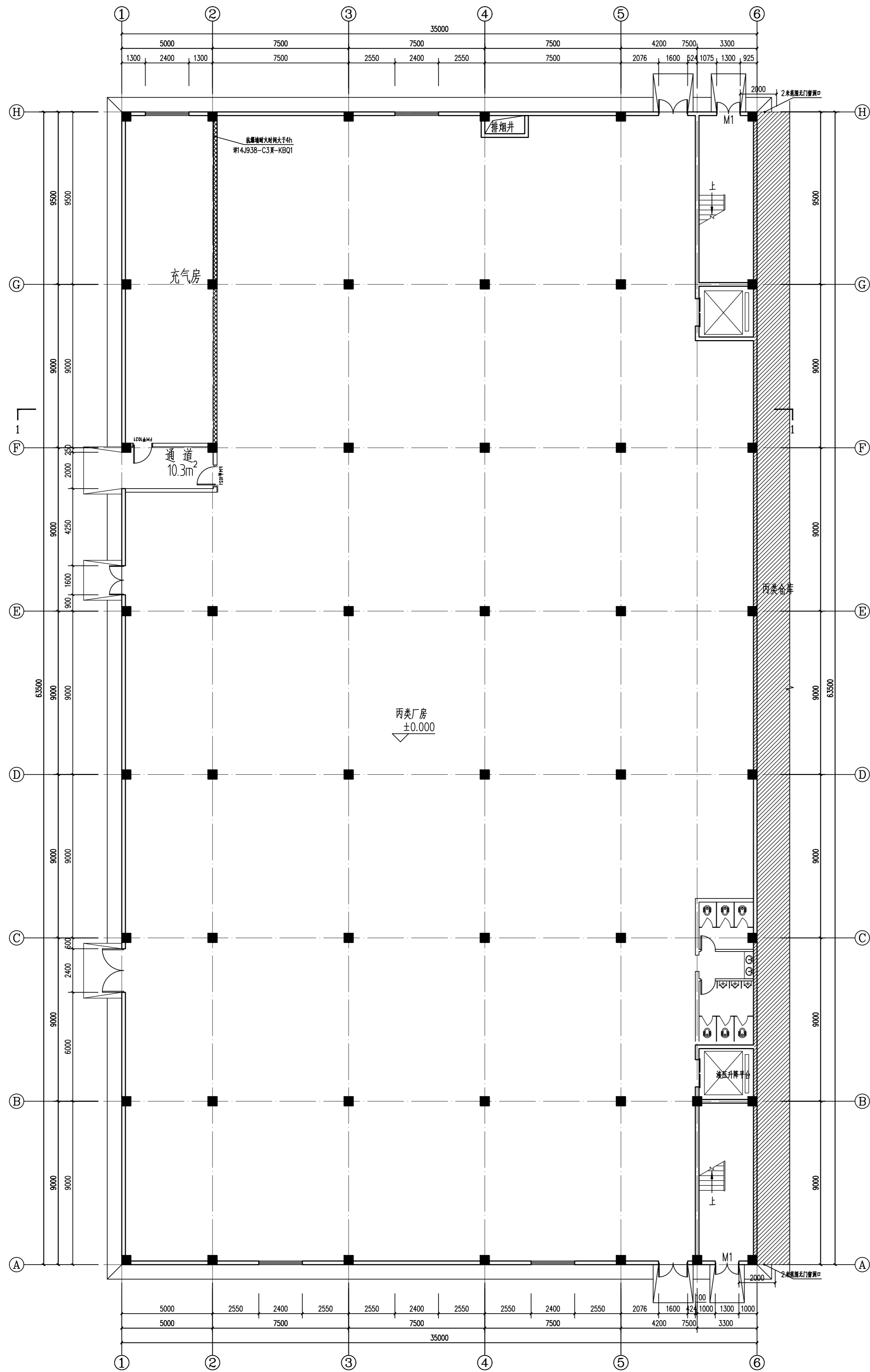
首层平面图 1:100
