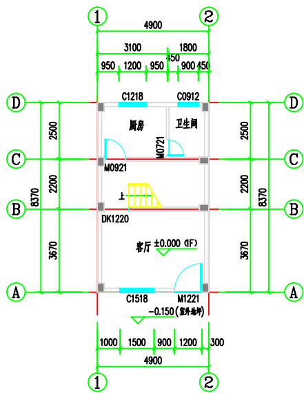
首层平面图 1:100
