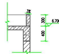
① 大样图 1:100
