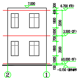
②-①轴立面图 1:100
