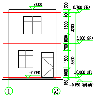
①-②轴立面图 1:100
