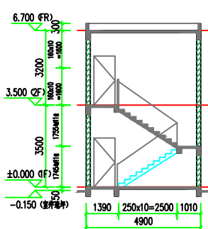
1-1剖面图 1:100
