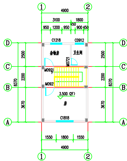
二层平面图 1:100
