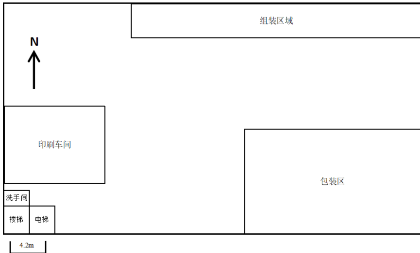
附图 2-3 项目车间平面布置图 (3F)
