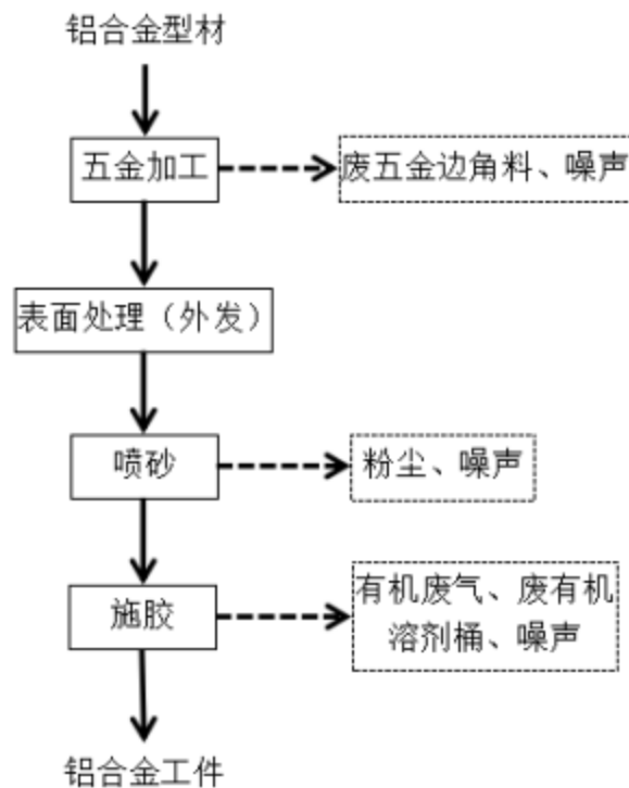
图4 铝合金工件生产工艺流程及产污分析图
