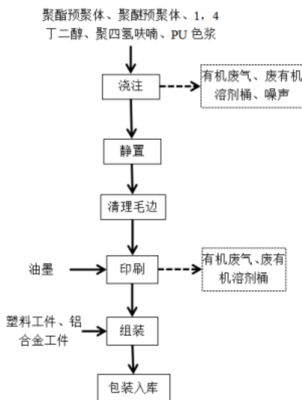
图 5 CPU 滑轮生产工艺流程及产污分析图
