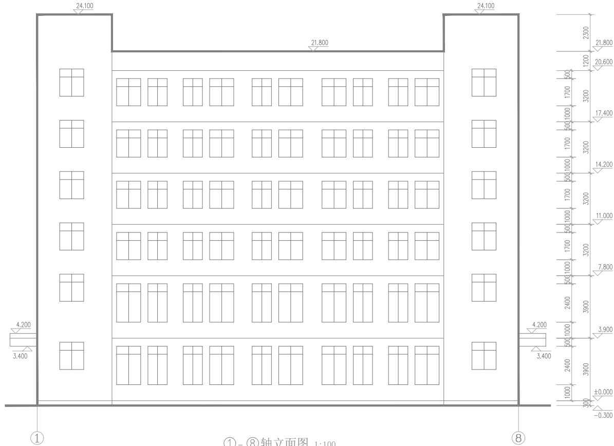
① - ⑧轴立面图 1:100
