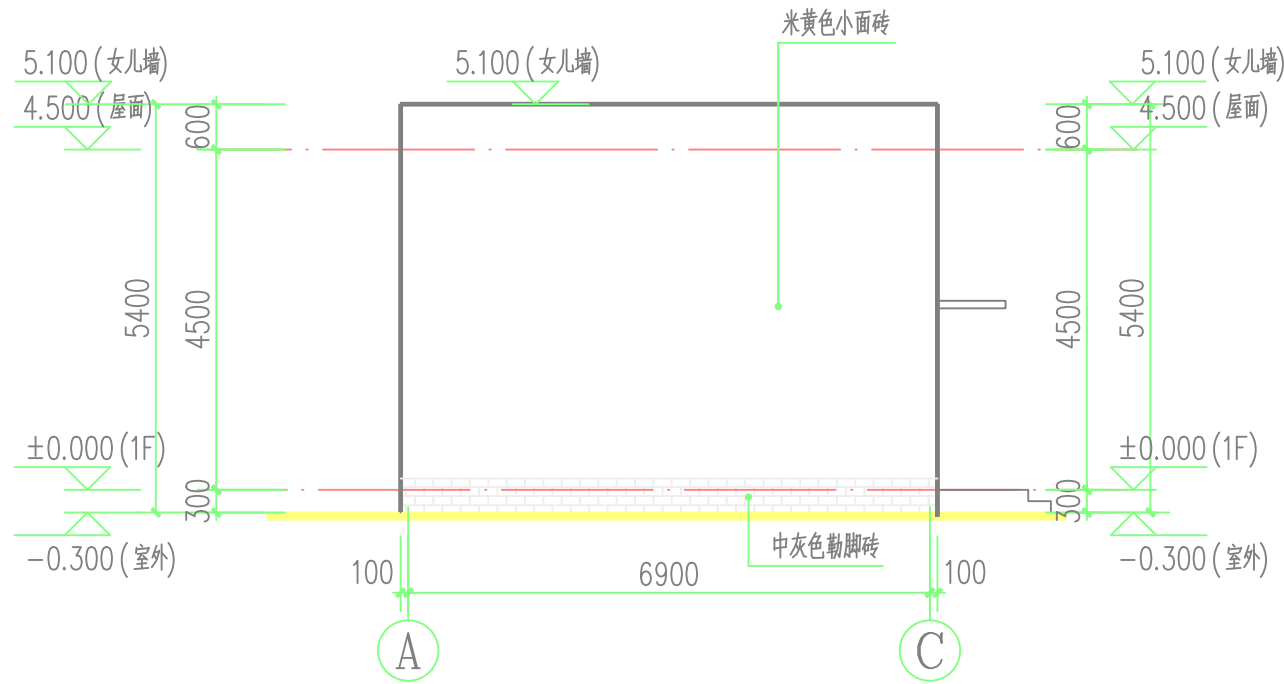
(A)-(C)立面图 1:100
