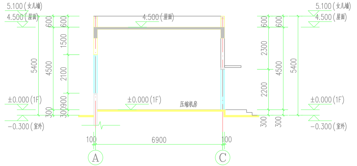
1-1剖面图 1:100
