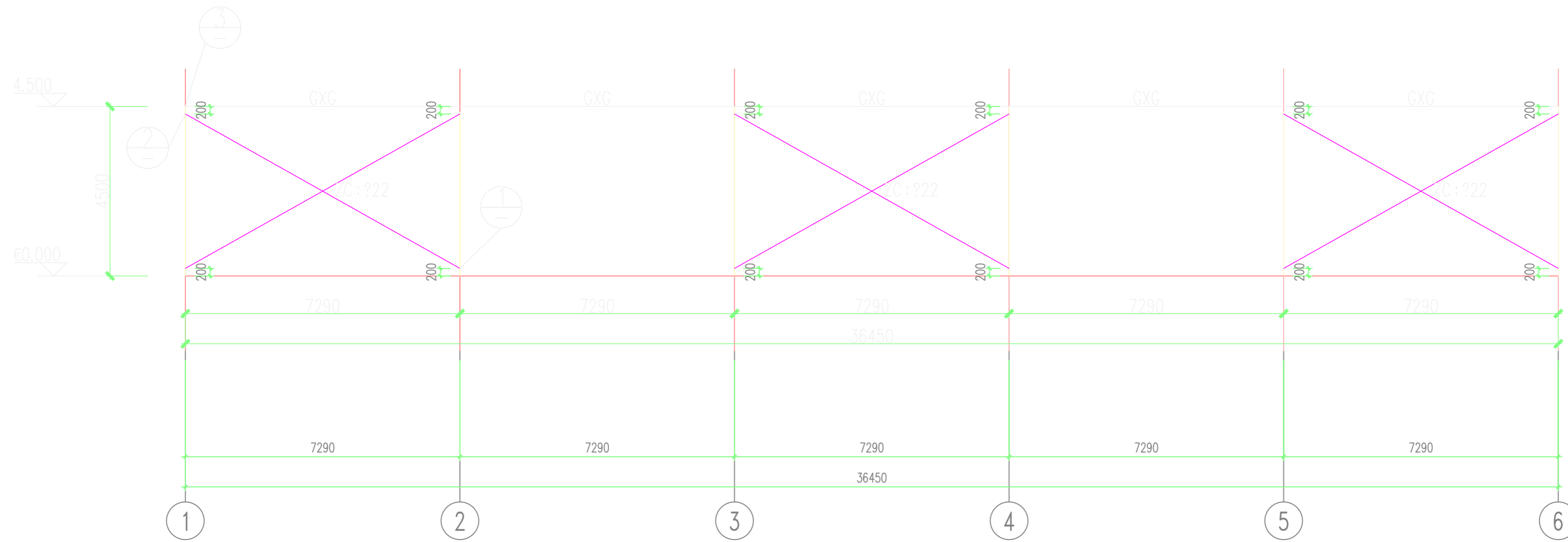
轴柱间支撑立面图 1:100
