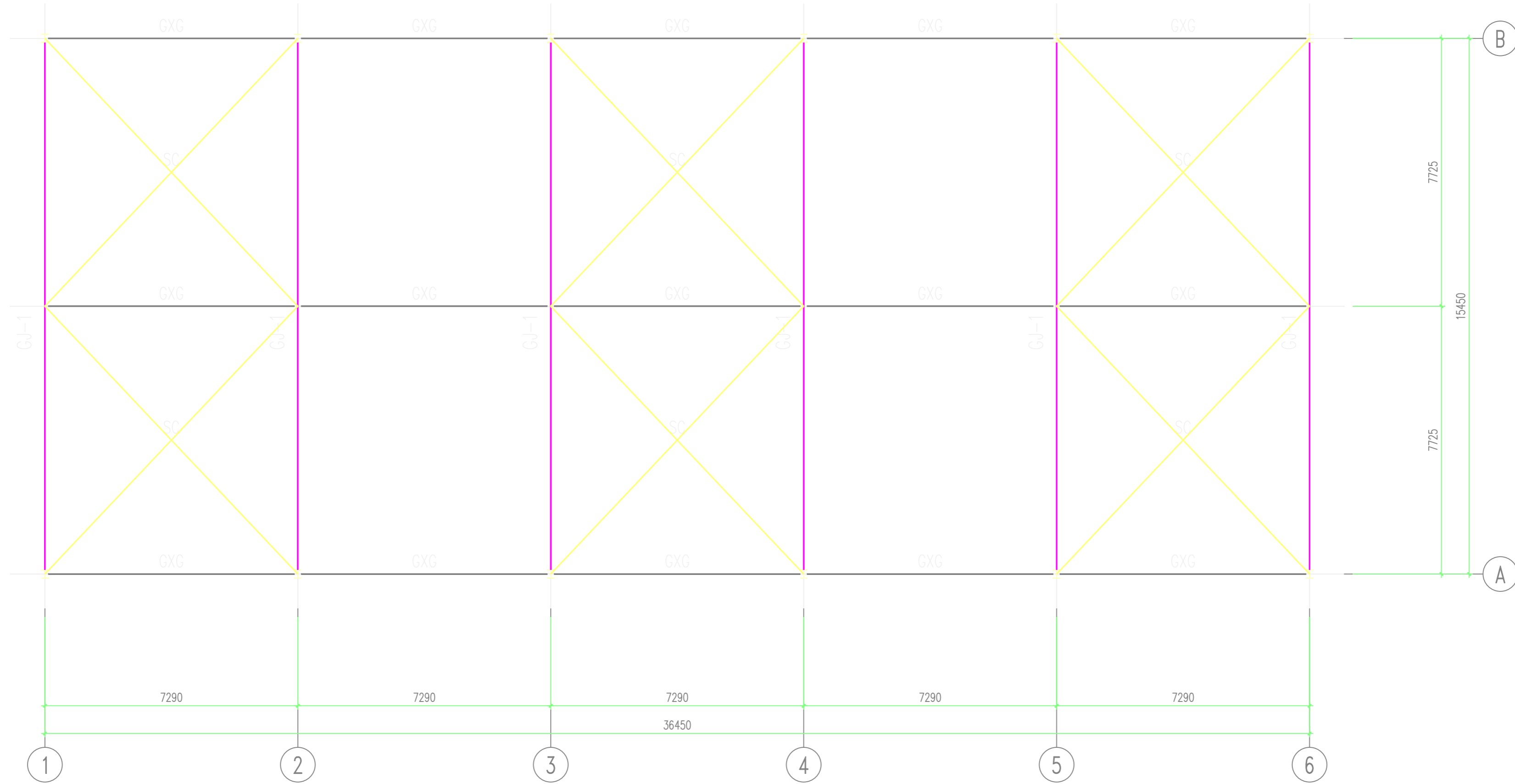
屋面支撑布置图 1:100
