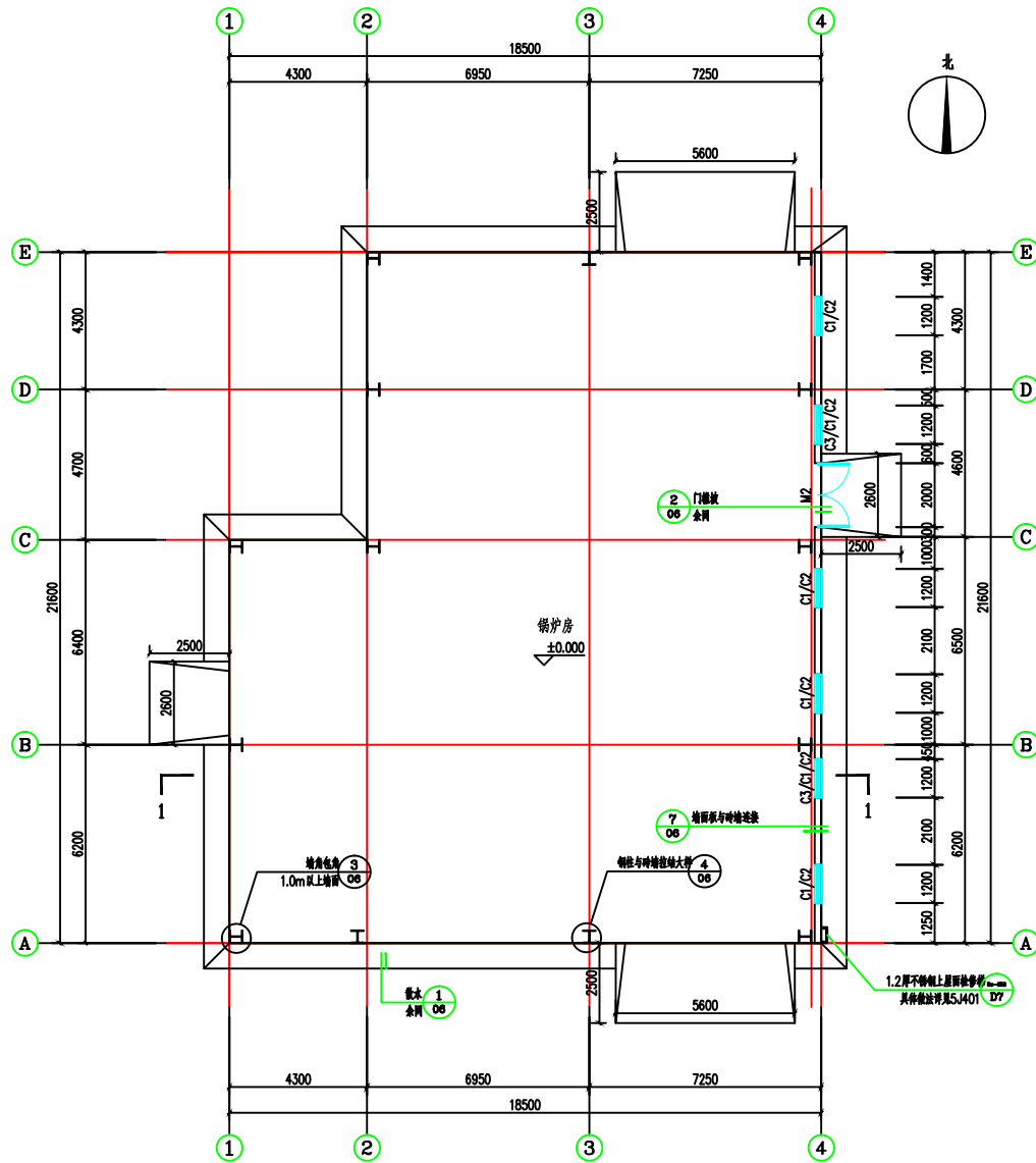
首层平面图 1:100
