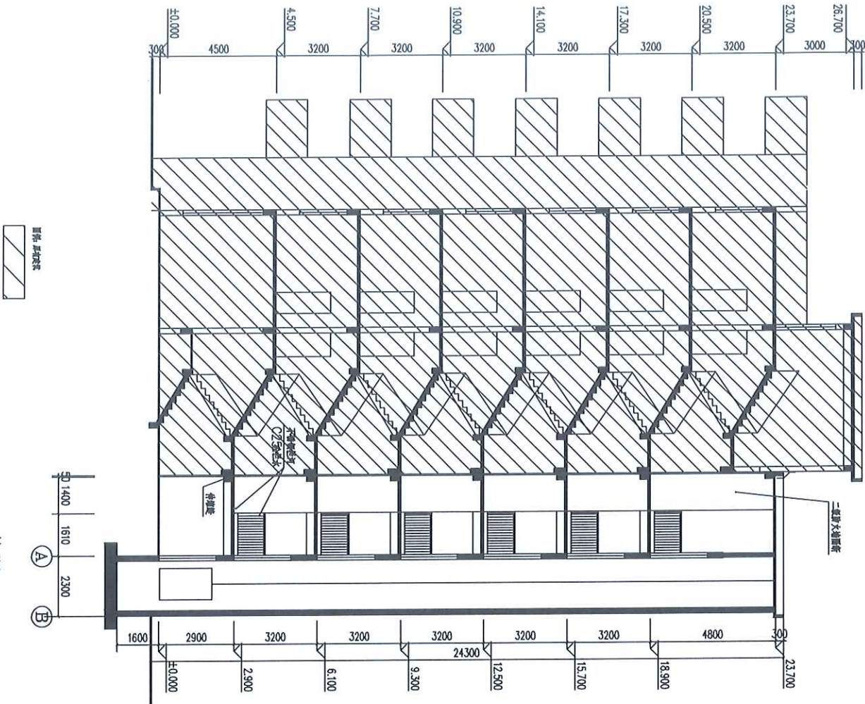
1-1剖面图 1:100
