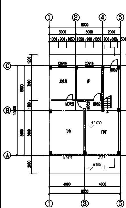
首层平面图 1:100
