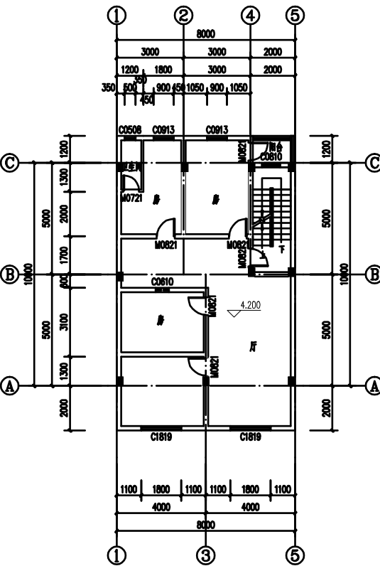
二层平面图 1:100
