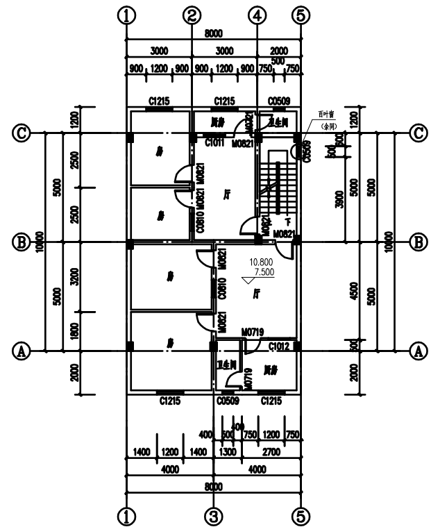
三至四层平面图 1:100
