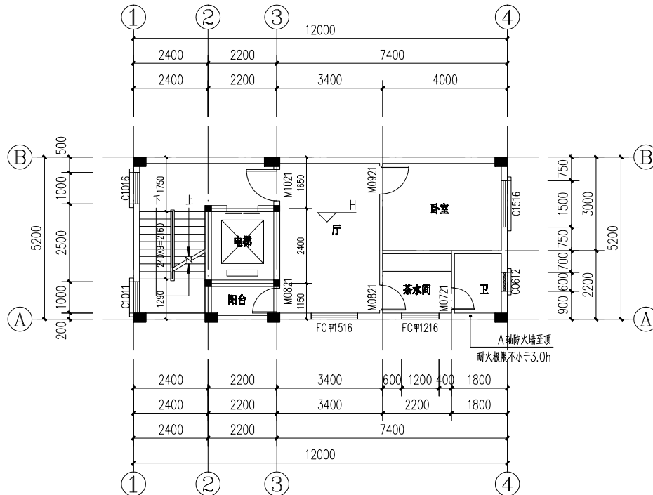
二至七层平面图 1:100
