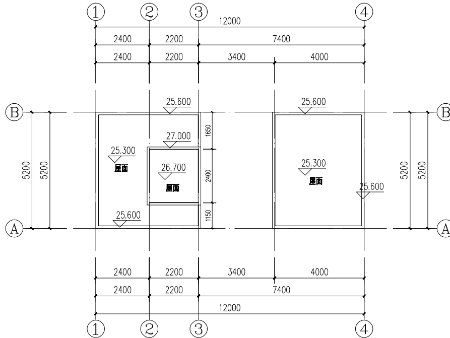
屋面平面图 1:100
