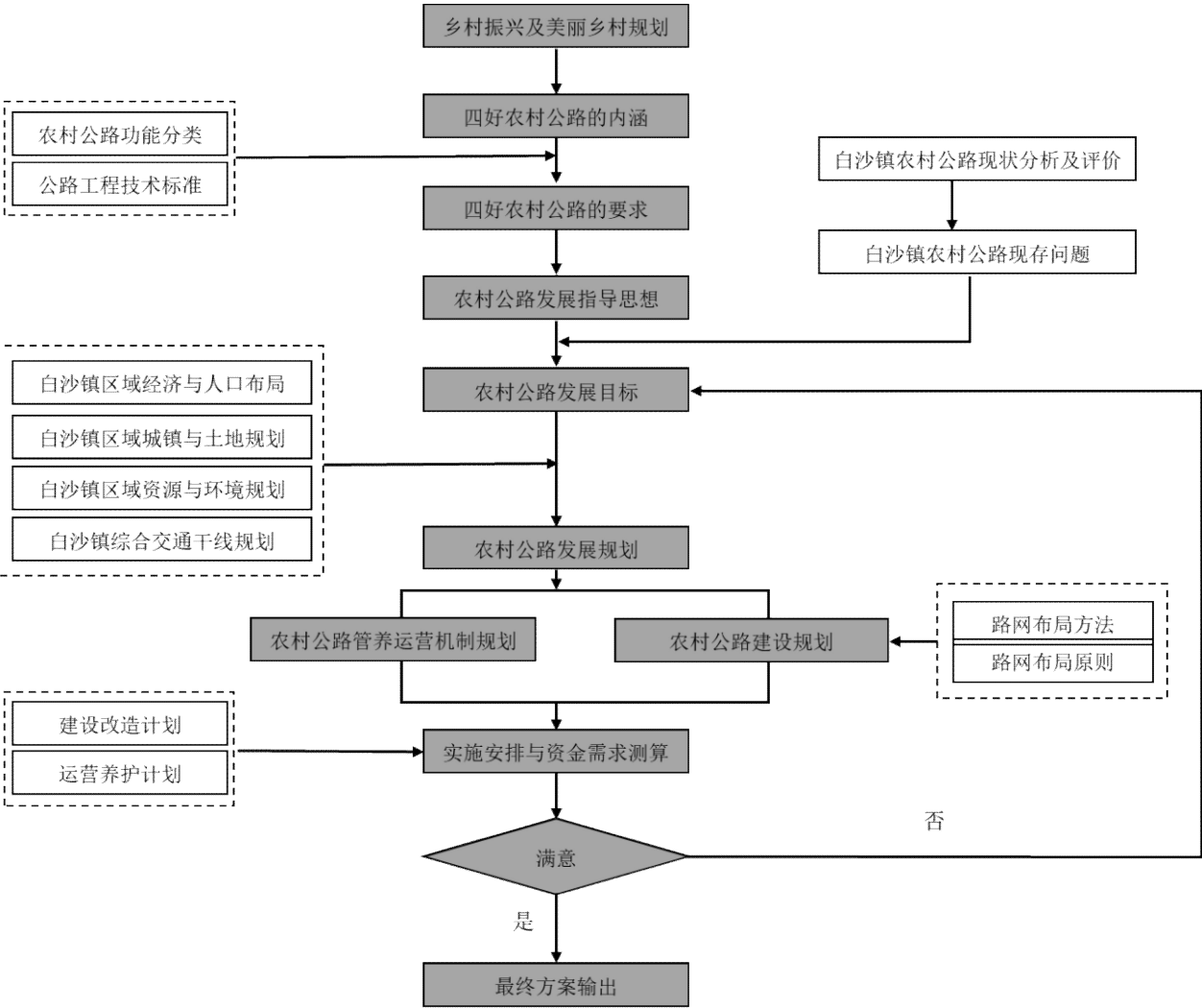
图 1-1 乡道、村道路网发展规划思路流程图
