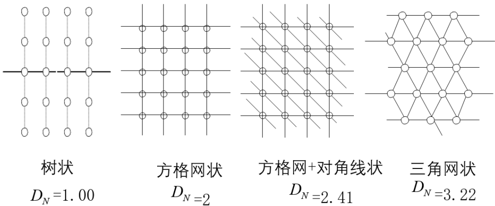
图 2-1 路网布局形式
