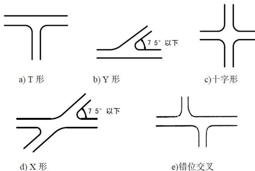
图 3-1 乡道、村道交叉口分类图
