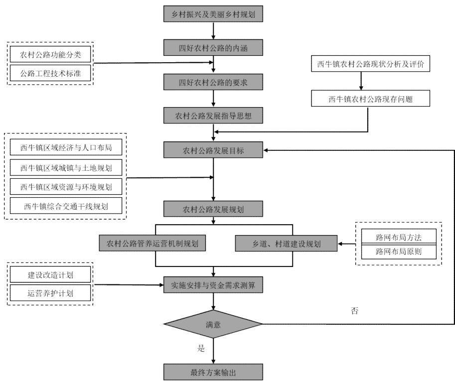
图 1-1 乡道、村道路网发展规划思路流程图
