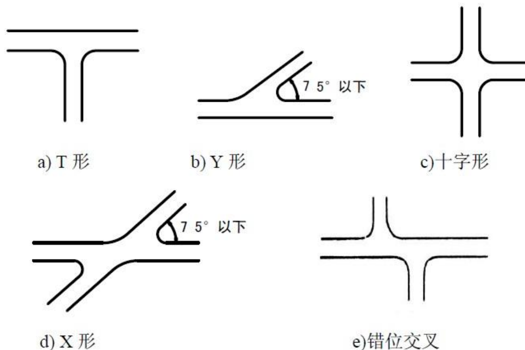
图 3-1 乡道、村道公路交叉口分类图
